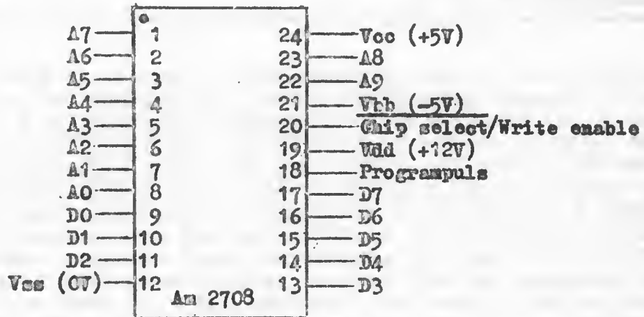
Fig. 1 Aansluitingen EPROM
